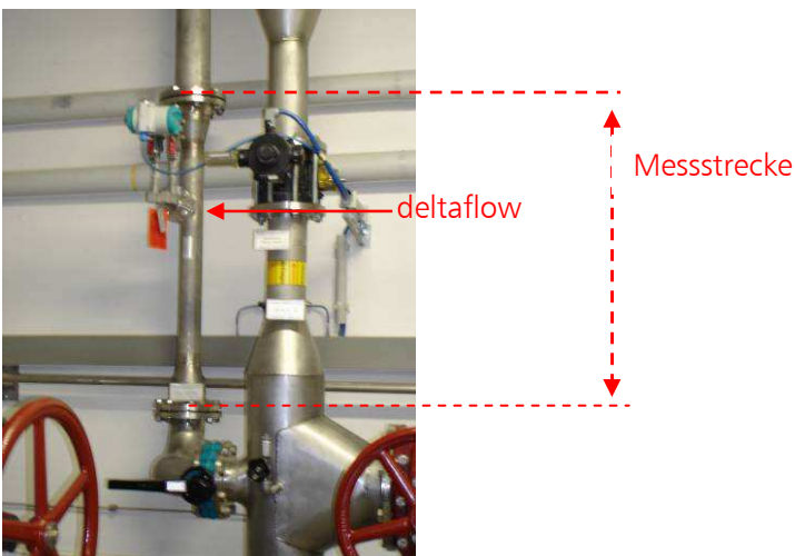
Abbildung 5 Beispiel deltaflow Messstrecke
